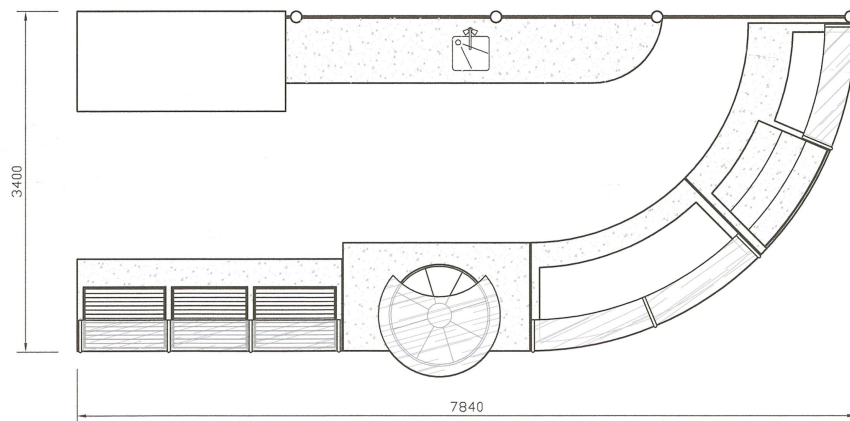
(Draufsicht)
