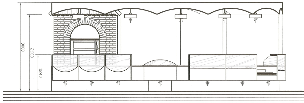
(Vorderansicht)
